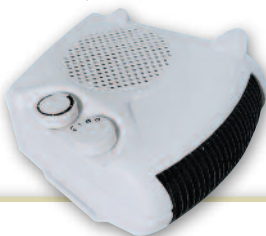
Ref. 29/248 CALEFACTOR TERMOVENTILADOR KA-5039 TRISTAR 2000 W. 3 funciones ajustables. Termostato regulable. Protección contra sobrecalentamiento. Luces piloto. Asa para transporte. 16,45€
