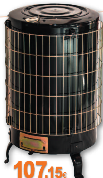
Ref. 36/155 ESTUFA DE LEÑA Nº4 ESMALTADA CON PARRILLA TALLER HNOS. CATALINA Salida horizontal Ø110 mm. Combustible sólo madera. Medida: alto: 615 mm Ø total 390 mm. Ø de carga 240 mm. Potencia máxima 14,5 KW. Marcado CE. 107,15€
